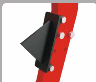
Clod - Lama spezzante
